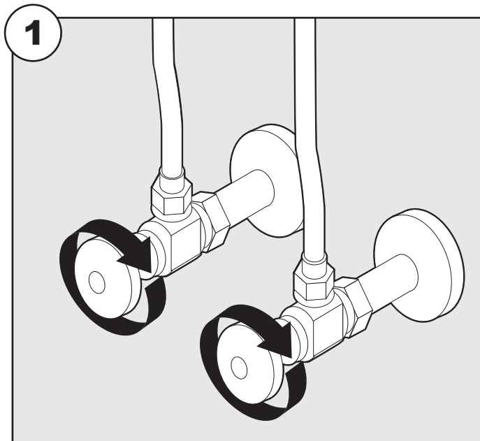
Turn off water supply. Remove existing faucet and water supply lines if necessary. Fermez l'alimentation d'eau. Enlevez le robinet existant et les conduites d'eau, si nécessaire. Cierra el suministro de agua. Quite el grifo existente y las líneas de abastecimiento de agua si es necesario.
