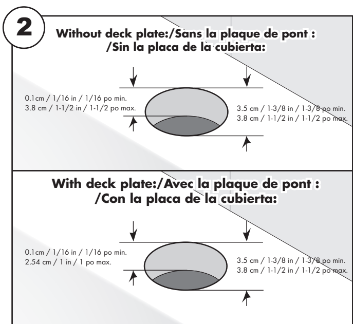
Check for proper thickness of sink. Vérifiez si l'évier est d'épaisseur correcte. Verifique el espesor apropiado del fregadero.
